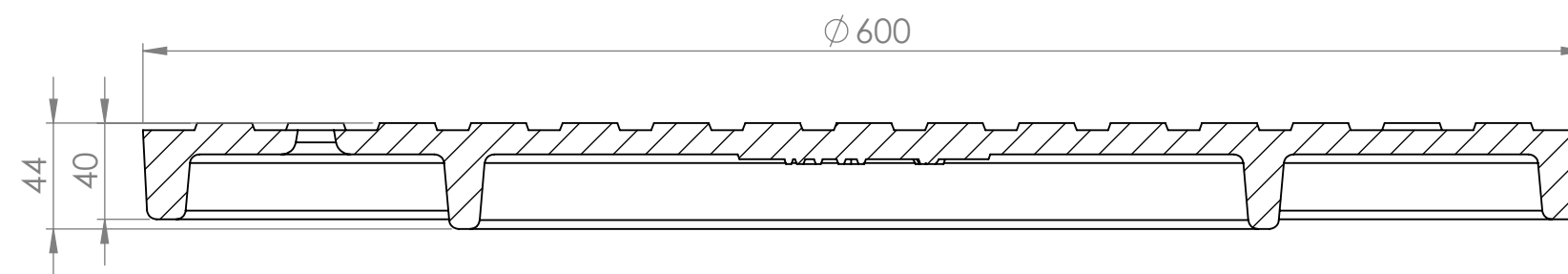
SECTION A-A
