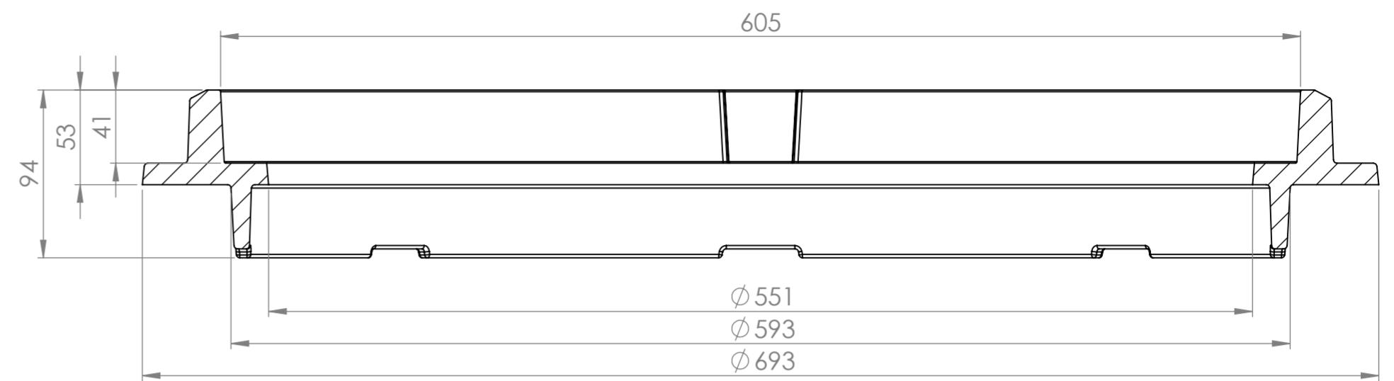
SECTION A-A
