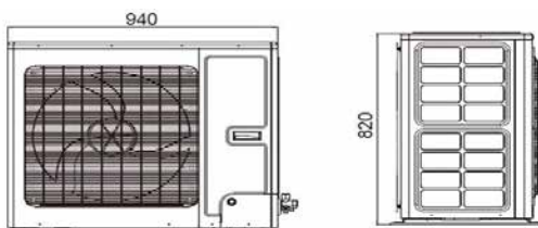
Yksikön mitat, mallit IGZAW12SNO3-1, IGZAW14SNO3-1, IGZAW14SNO3-1
