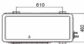
Yksikön mitat, mallit IGZAW12SNO3-1, IGZAW14SNO3-1, IGZAW14SNO3-1
