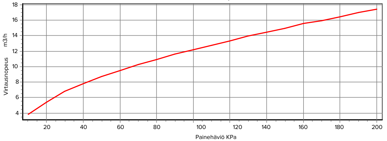
Painehäviö/virtausnopeus
